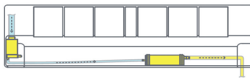
Watersensor verticaal en pomp horizontaal in het binnentoestel.
