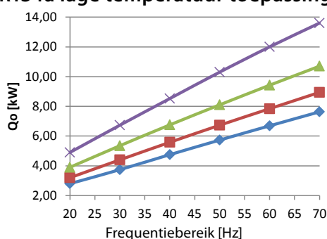
R134a lage temperatuur toepassingen
