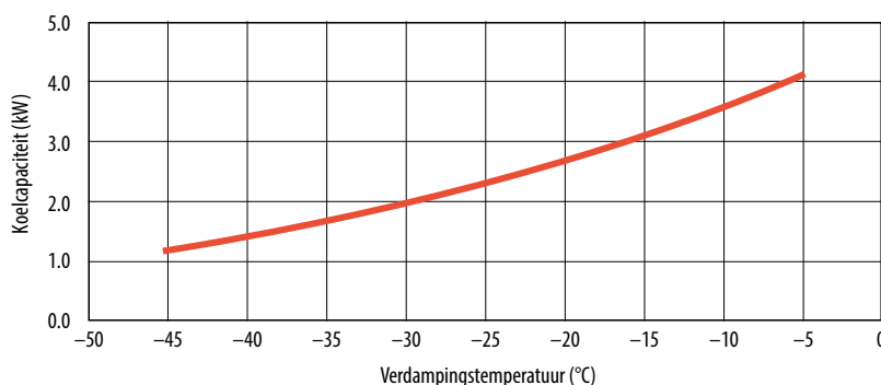
Capaciteiten in functie van T 0 bij 65 Hz
