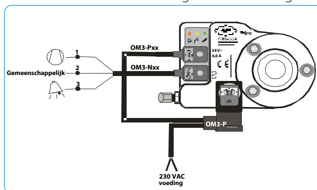
Schematische voorstelling OM3 aansluiting
