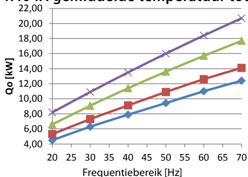
R404A gemiddelde temperatuur toepassingen
