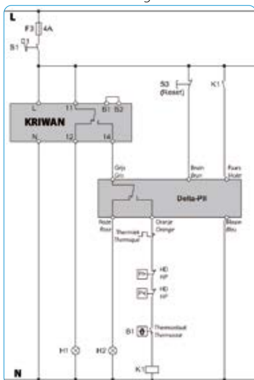
Schematische voorstelling Delta PII aansluiting
