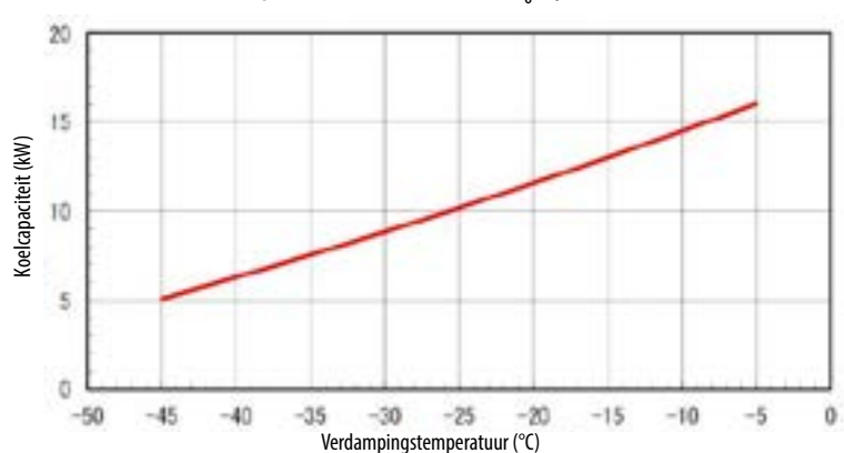
Capaciteiten in functie van T o bij 65 Hz
