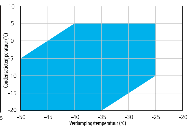
CO 2 werkingsbereik HGX4 CO 2 Oververhitting zuiggas = 10 K
