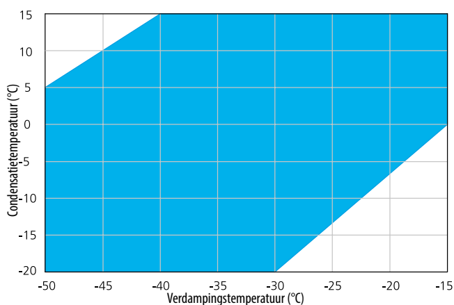
CO 2 werkingsbereik HGX12e CO 2 - HGX22e CO 2 - HGX34e CO 2 Oververhitting zuiggas = 10 K
