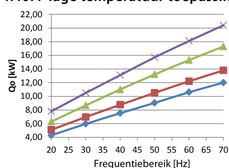
R407F lage temperatuur toepassingen
